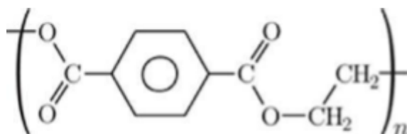
Fig. 18 : Molécule de polyéthylène téréphtalate
