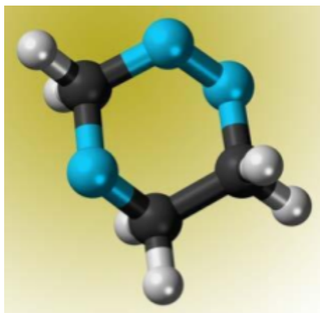
Fig. 55 : Structure tridimensionnelle du 1,2,4 trioxane
